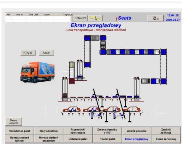
Rys6. Ekran linii montażu siedzeń
