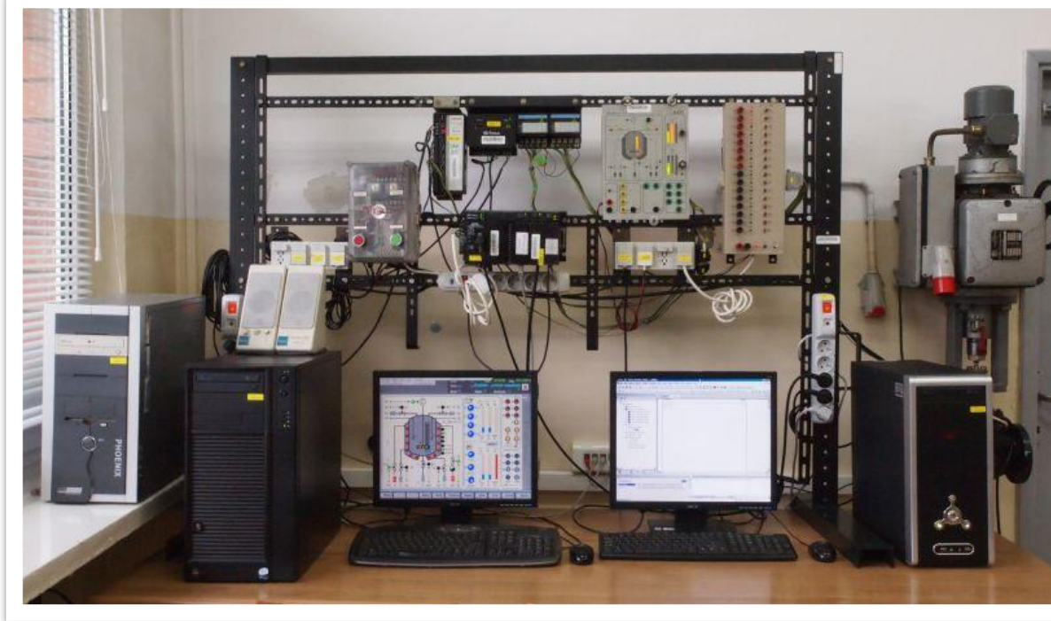
Rys1. Widok stanowiska laboratoryjnego
